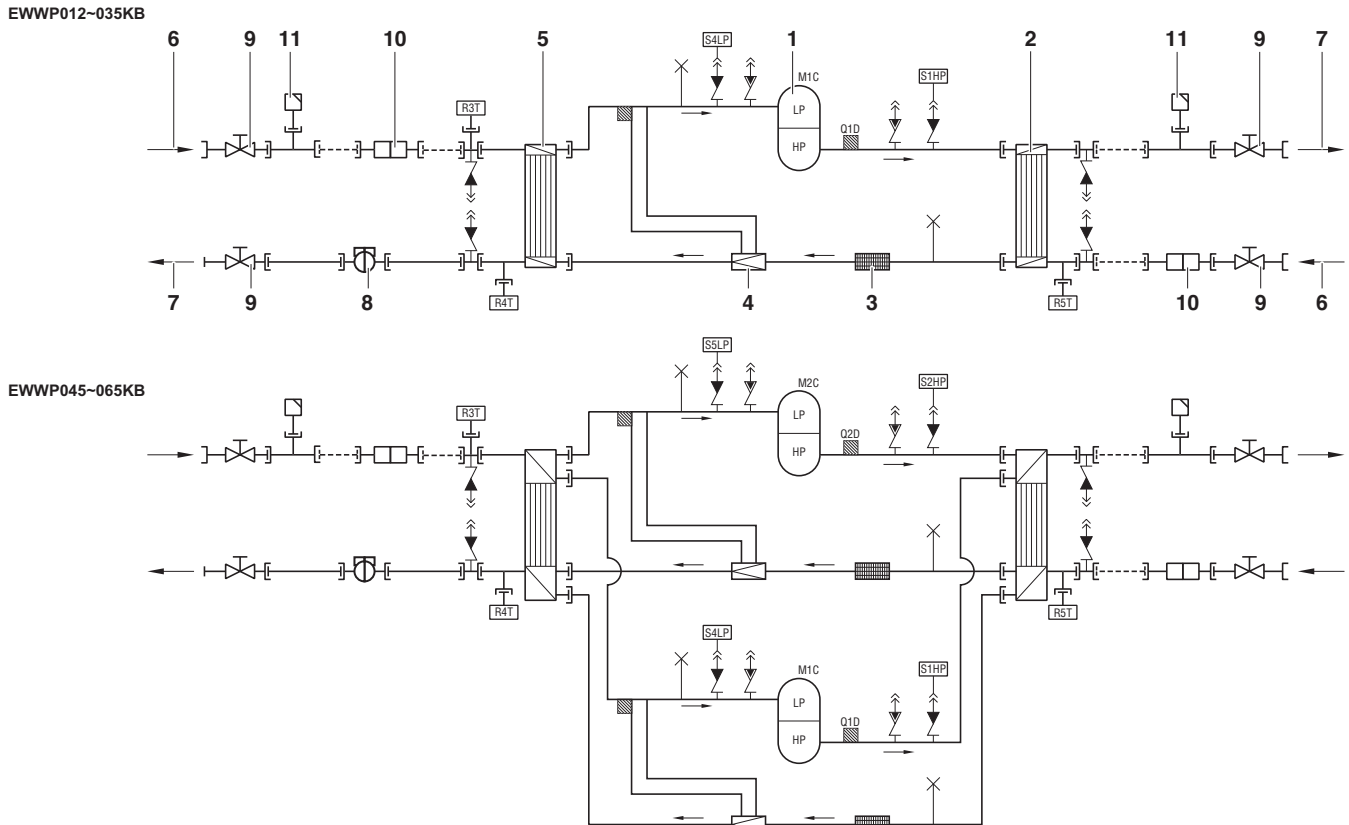
Figura – Diagramă funcțională
